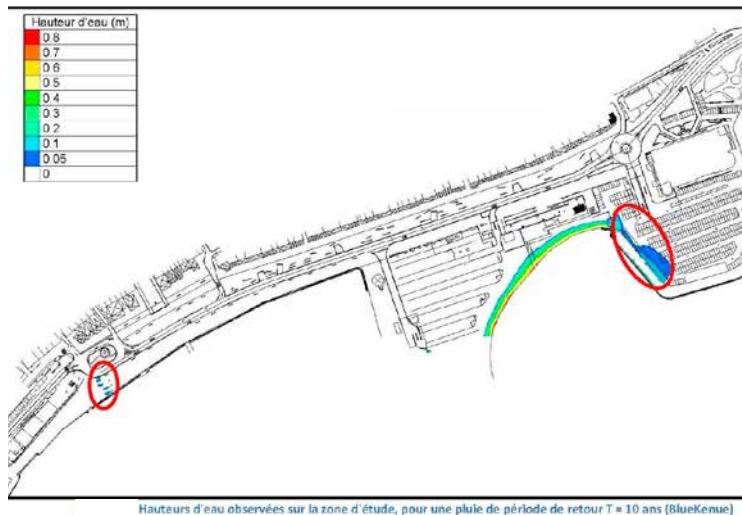
Hauteurs d'eau observées sur la zone d'étude, pour une pluie de période de retour T = 10 ans (BlueKenue)
